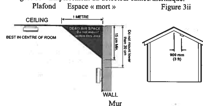
Figure 3i – Emplacement du détecteur fumée/thermique.
